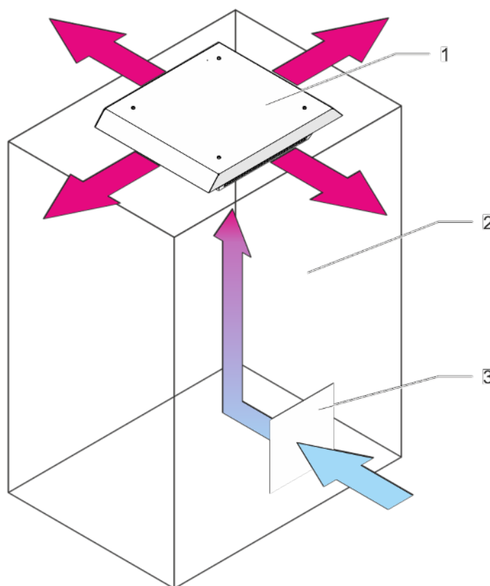
Fig. 3: Descrizione del funzionamento del ventilatore con filtro da tetto PTF (esempio)
