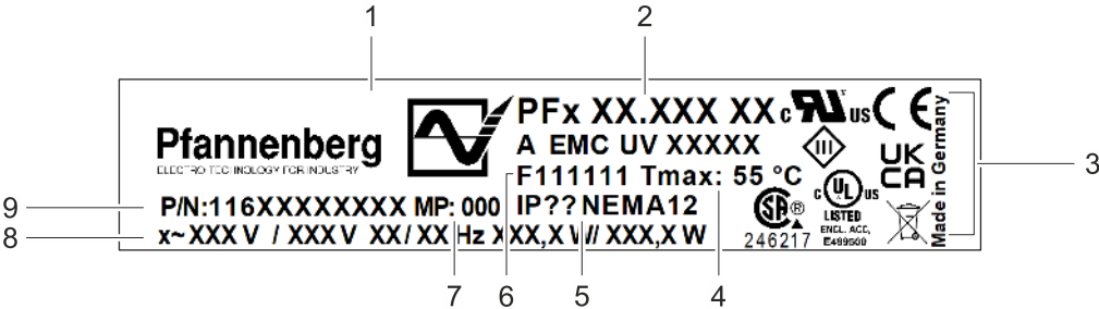
Abb. 5: Typenschild (Beispiel)
