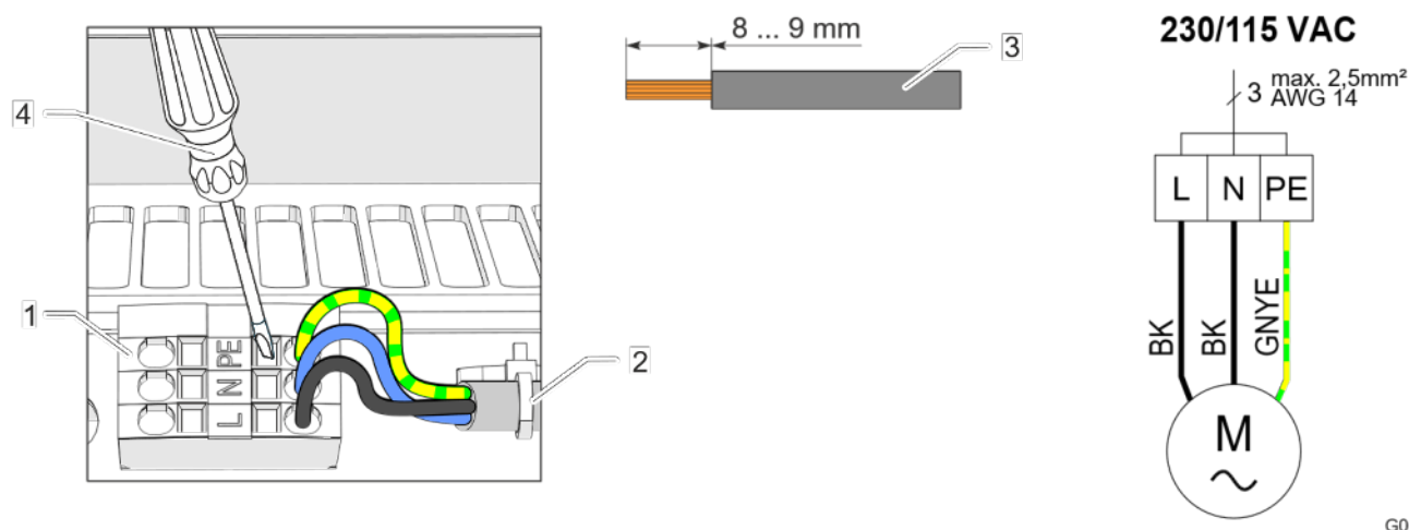
Рис. 10: Подключение питания PTF 6х.xxx
