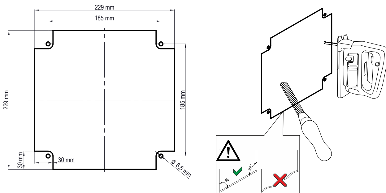
Abb. 9: Montageausschnitt / Montage
