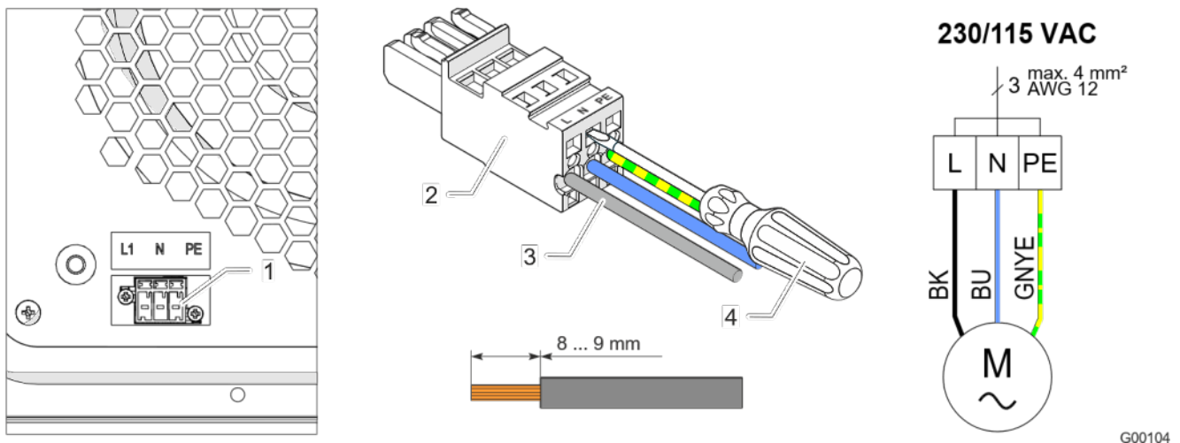
Fig. 11: Conector de alimentación - PTF1200
