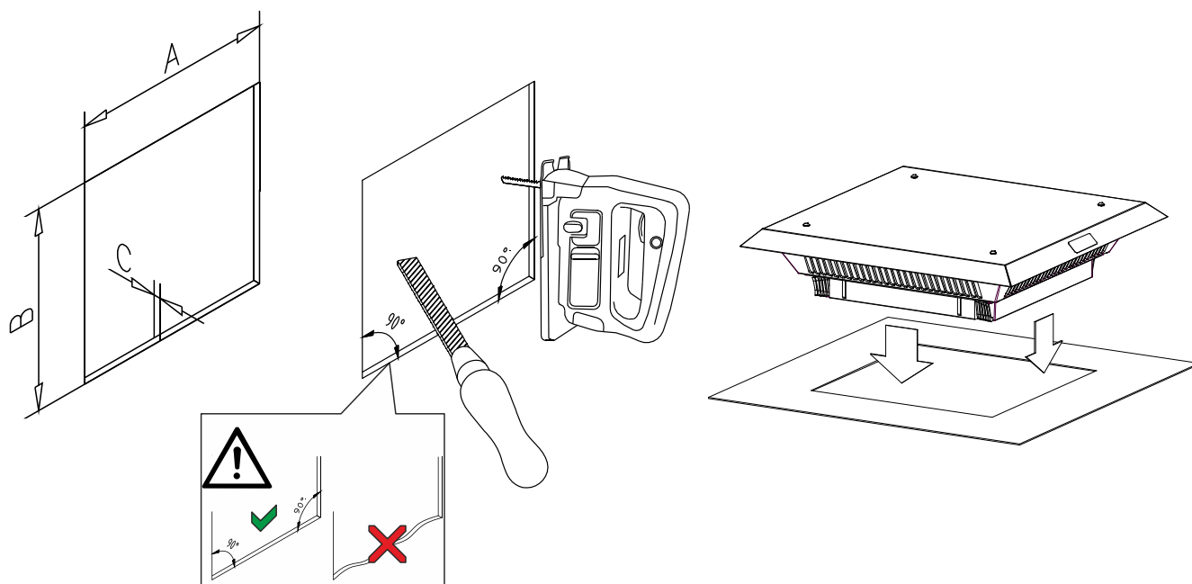
Abb. 8: Montageausschnitt / Montage
