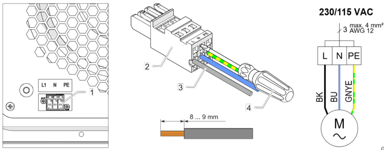
Fig. 11 : fiche de raccordement secteur PTF 1200
