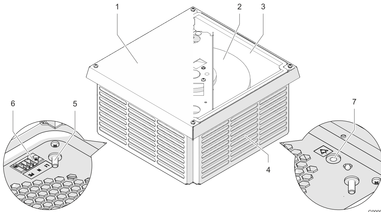
Abb. 2: Geräteaufbau PTF 1200
