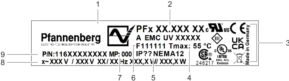
Fig. 5: Placa de características (ejemplo)
