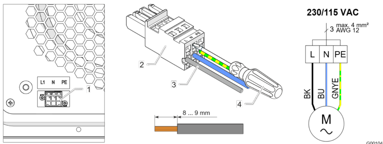
Fig. 11: Connettore di rete PTF1200
