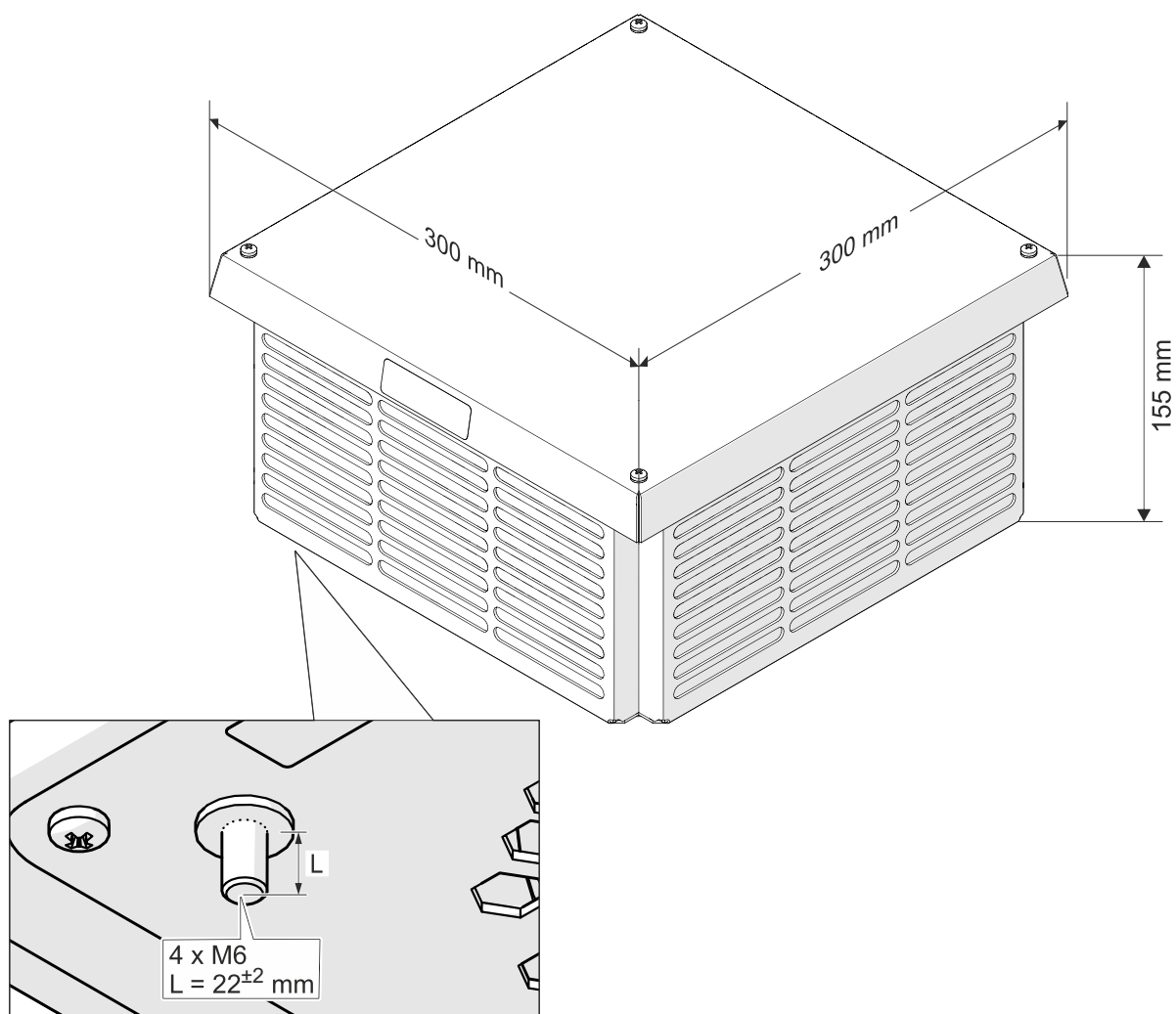
Abb. 7: Abmessungen
